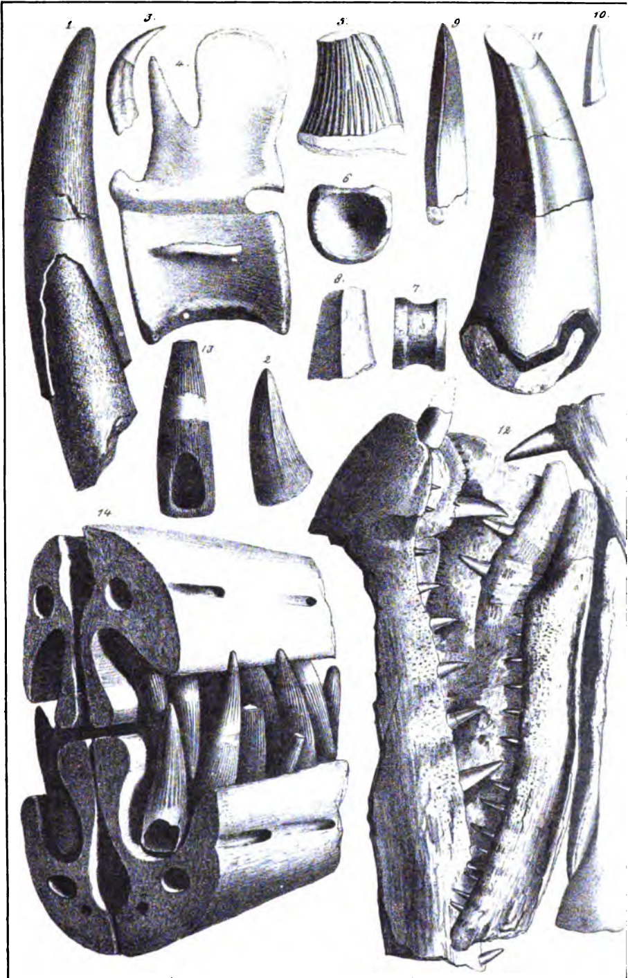
Quenstedt, Jura.
